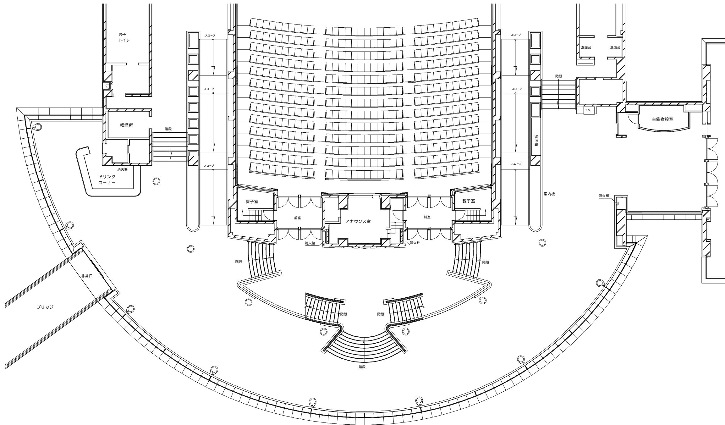
福井県立音楽堂 大ホール ホワイエ詳細図 縮尺 1 / 2 0 0
